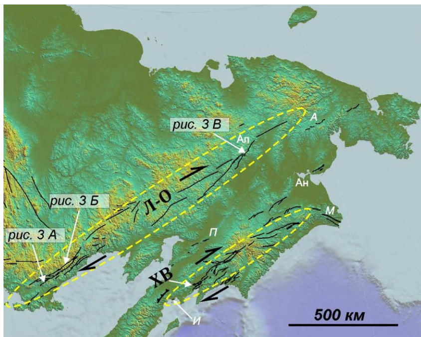
Рис. 2. Схема активных разломов СВ Азии по данным дешифрирования снимков КН-9 ( http://earthexplorer.usgs.gov/ ). Л-О – Ланково-Омолонская зона, ХВ – Хатырско-Вывенская зона. А – Амгуэмская впадина, М – Мейныпильгынский хр., И – п-ов Ильпыр, П – Пенжинский хр., Ан – Анадырская низменность, Ап – Анадырское плоскогорье.
