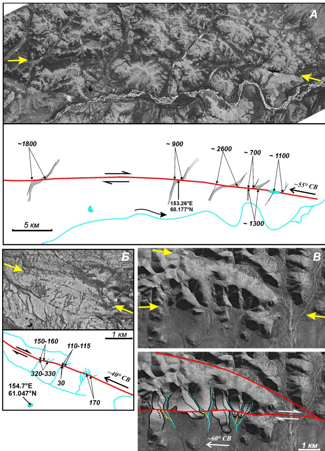
Рис. 3. Правосторонние смещения вдоль разломов Ланково-Омолонской зоны (Кожурин, 2012). А, Б – в южной части зоны (координаты центров рисунков примерно 153.343^\circ в.д., 60.277^\circ с.ш. и 154.74^\circ в.д., 61.04^\circ с.ш., соответственно), цифры внизу - амплитуды смещений, м; В – в северной части зоны (координаты центра 171.565695^\circ в.д., 66.026071^\circ с.ш.), красные линии – активные разлома, черные точечные – линии водоразделов. Положение рисунков см. на рис. 3.1.
