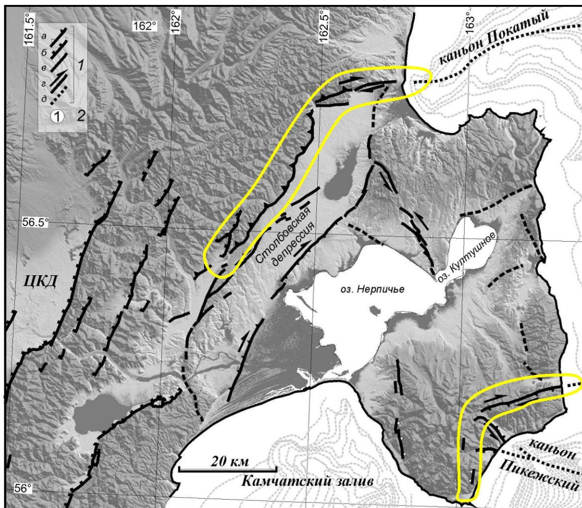
Рис. 4. Активные разломы полуострова Камчатский. 1 – разломы: взбросы (а), сбросы (б), неопределенной кинематики (в), сдвиги и со сдвиговой компонентой (г) и их возможные подводные продолжения (д); 2 – номера разломов (см. текст); 3 – примерное положение канав (см. текст). Основа рисунка – SRTM data V3, http://srtm.csi.cgiar.org (Jarvis et al., 2006). По (Kozhurin, 2007a; Кожурин, Пинегина, 2011; Kozhurin, Pinegina, 2011a, 2011b; Кожурин и др., 2014, в печати) с дополнениями
