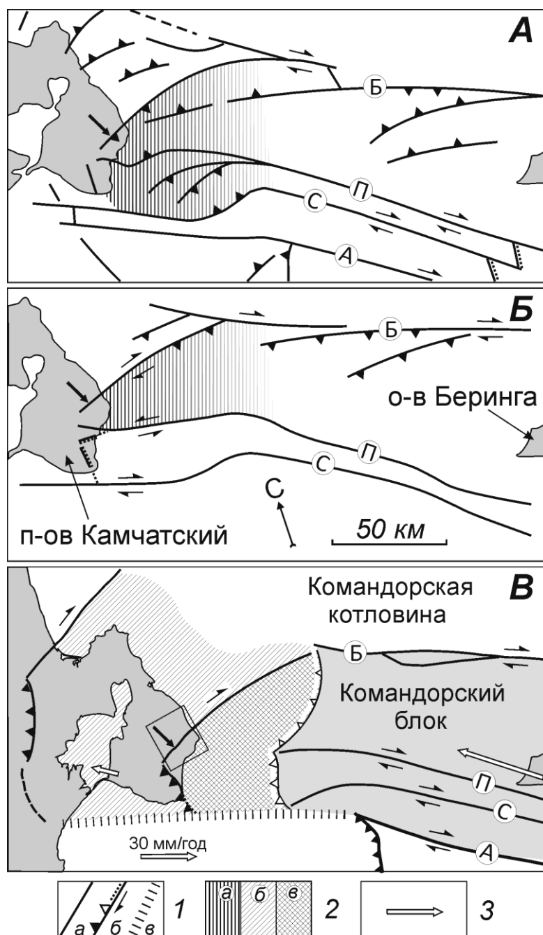
Рис. 5. Модели коллизионного взаимодействия Алеутской и Камчатской островных дуг: А – по (Gaedike et al., 2000), Б – по (Баранов и др. 2010), В – по (Кожурин и др., 2014, в печати). 1 – активные разломы основные (а), (б) – взбросовое или надвиговое (треугольники), сдвиговое (стрелки) и сбросовое (штрихи) направление движений по разломам (незалитые символы соответствуют предполагаемому направлению движений), край погруженной части Тихоокеанской плиты (в); 2 – фронтальная часть единого Командорского блока (а) (на А и Б) и блоки западной (основной) части п-ова Камчатский (б) и его юго-восточной части (в) (на В); 3 – векторы смещений пунктов GPS (на В): западная стрелка – пункт в пос. Крутоберегово, восточная – пункт в пос. Беринга. Подводные разломы Командорского сегмента Алеутской дуги на В показаны по (Селиверстов и др., 1995). Буквы в кружках – названия разломов: Б – Беринга, П – Пикеж, С – Стеллера, А – Алеутский (по оси глубоководного желоба). Черная стрелка на А, Б и В указывает на разлом 2-й Перевальный
