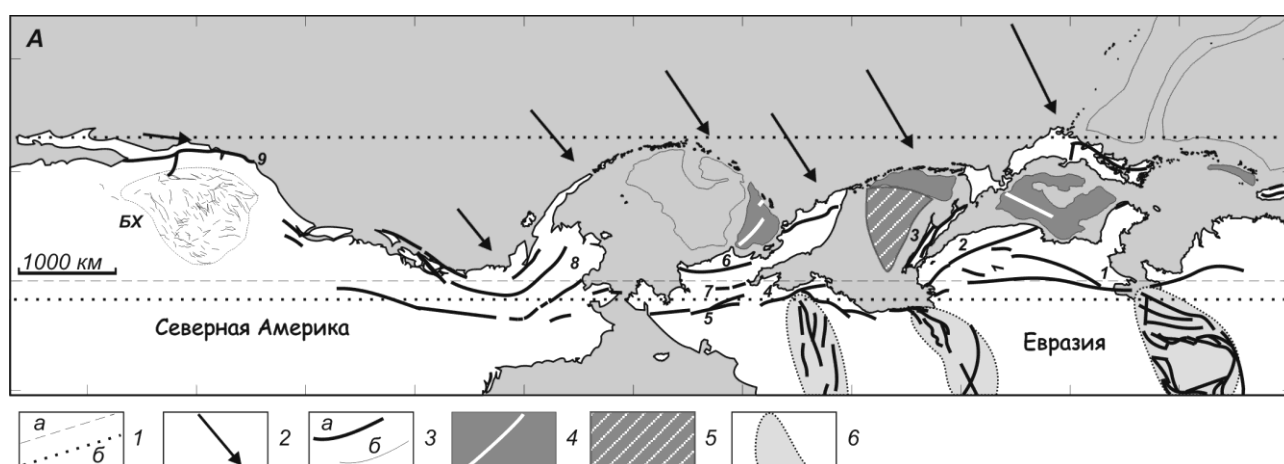
Рис. 1. Позднекайнозойский Тихоокеанский пояс (по (Kozhurin, 2004) с изменениями и дополнениями). 1 – дуга большого круга, описывающая положение на сфере Американской и Азиатской окраин Тихого океана (а) и примерные ограничения структур пояса (б); 2 – векторы относительного движения Тихоокеанской плиты относительно Северной Америки и Евразии; 3 – основные правосдвиговые активные разломы пояса (а), сбросы Провинции Бассейнов и Хребтов (б); 4 – задуговые впадины растяжения с новообразованной океанической корой и оси спрединга в них; 5 – участки с утоненной континентальной корой; 6 – примерные контуры внутриконтинентальных подвижных поясов. Цифры – правосдвиговые разломы: 1 – Танлу, 2 – Центральный Сихоте-Алиньский, 3 – Сахалинский, 4-5 – Ланково-Омолонская зона, 6 – Хатырско-Вывенская зона, 7 – предполагаемая разломная зона Пенжинского хребта, 8 – Денали, 9 – Сан-Андреас. БХ – Провинция Бассейнов и Хребтов.
