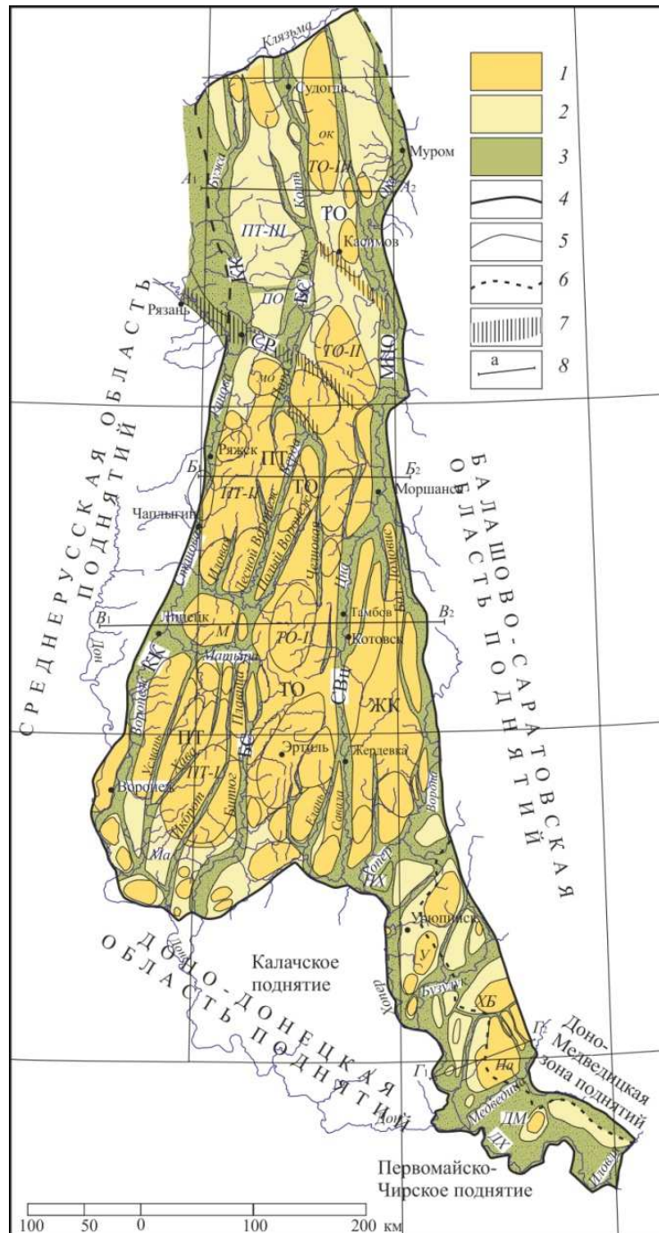
Рис. 3. Современный структурный план Окско-Донского прогиба [Корчуганова, Соколов, Загубный, 2012]
