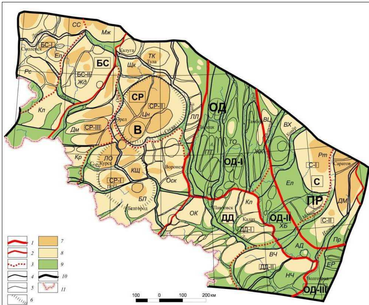
Рис. 1. Неотектоническое районирование территории Воронежского кристаллического массива [Корчуганова, Соколов, Загубный, 2012]
