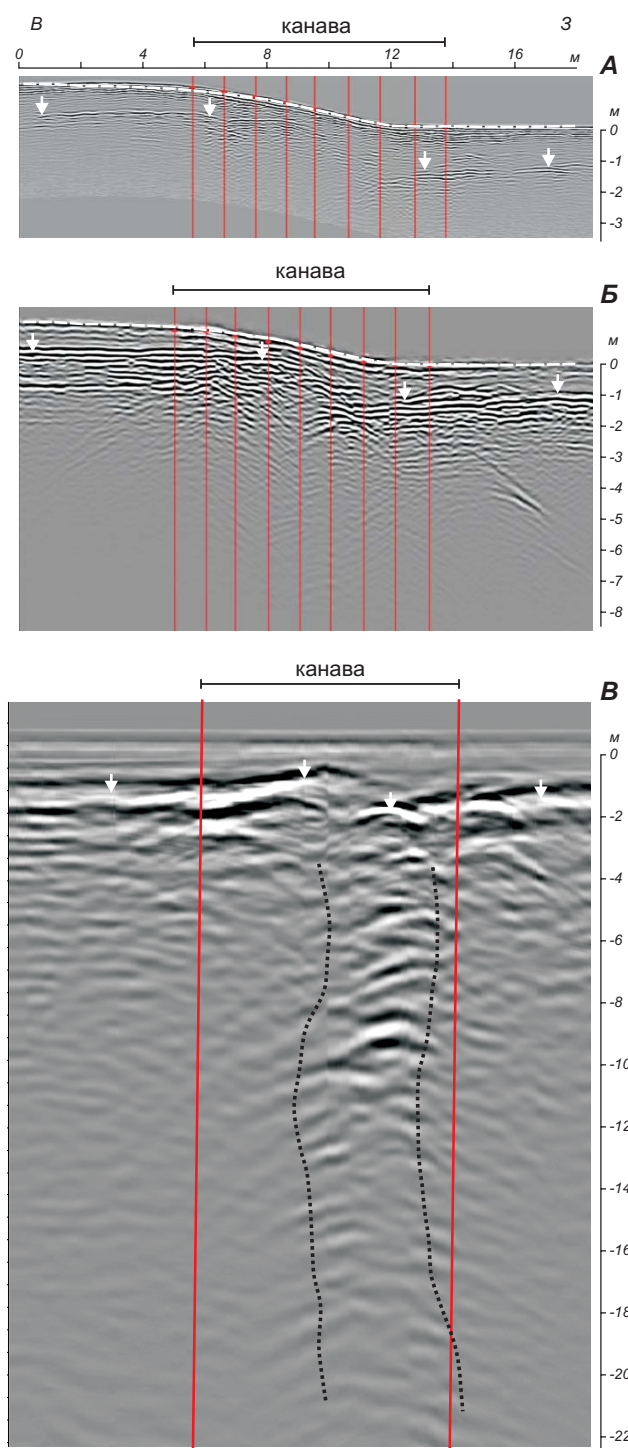
Рис. 9. Георадарные профили, пройденные вдоль южной стенки канавы вкрест разломного уступа. А — с антенной АБ 700, Б — с антенной АБ 250, В — с антенным блоком АБД «Тритон». Соотношение вертикального и горизонтального масштабов — 1:1. Вертикальные сплошные линии на А и Б проведены через 1 м, на С — ограничивают канаву. Белая пунктирная линия — часть гипсометрического профиля, показанного на рис. 8А. Вертикальные стрелки показывают положение поверхности валунно-галечных отложений горизонта 1 (рис. 8Б). Точечные линии на рис. 8В — примерные ограничения зоны, в которой находится плоскость разлома (интерпретация). Радарограммы на рис. 8А и рис. 8Б привязаны к гипсометрическому профилю, радарограмма на рис. 8С показана без привязки.
