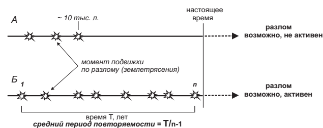
Рис. 2. Принципиальная схема возможных соотношений периода повторяемости подвижек и возраста последней подвижки по активному и неактивному разломам (пояснения в тексте).
