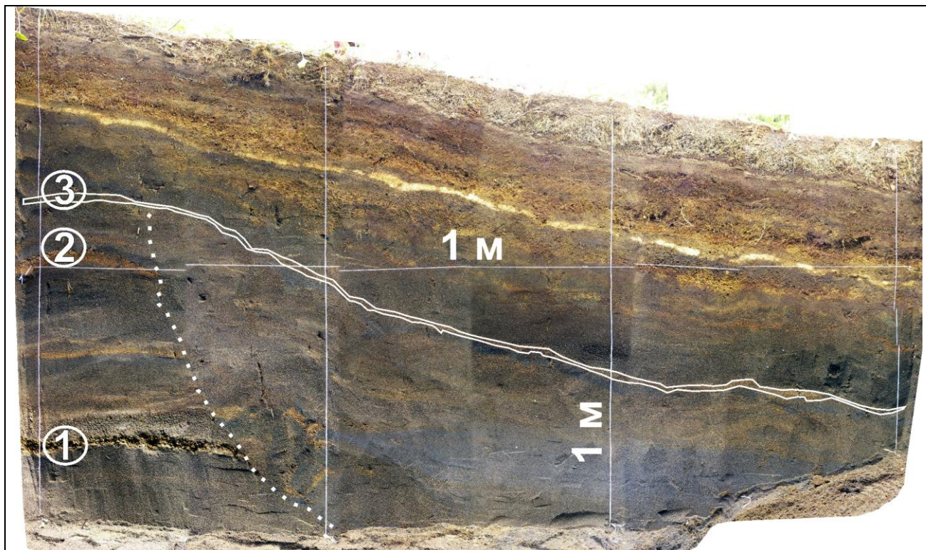
Рис.3. Вскрытый в стенке канавы погребенный уступ размыва №2 (точечный пунктир). Канавка заложена перпендикулярно простиранию берегового вала, море находится справа. Цифрам 1, 2, 3 соответствуют горизонты тефры возраста 2650 ^{14}\text{C} , 2500 ^{14}\text{C} , 2400 ^{14}\text{C} лет. Белой линией обведен горизонт тефры 3, перекрывающей уступ. Возраст уступа 2450 \pm 50 ^{14}\text{C} лет.
