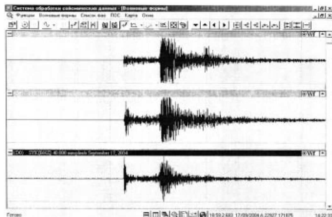
Рис. 1. Волновая картина Емвинского землетрясения, зарегистрированного с/станцией "Сыктывкар"
