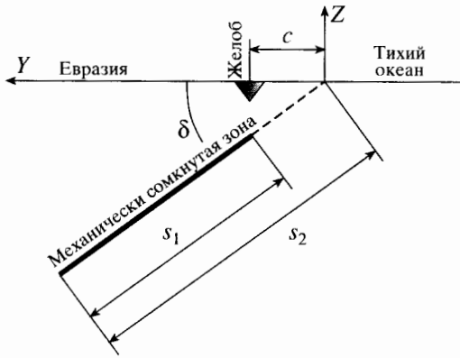
Рис. 3. Схема зоны субдукции.
