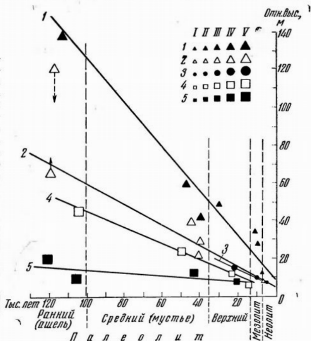
Рис. 2. Графики связи относительной высоты расположения и возраста приречных стоянок каменного века (графики врезания рек). Составлены по материалам А. П. Окладникова, В. А. Ранова, А. А. Никонова, С. Л. Троицкого (Средняя Азия, Монголия), В. П. Любина, В. М. Муратова (Кавказ), А. Г. Медоева (Казахстан), И. К. Ивановой, П. И. Борисовского (Русская равнина)
